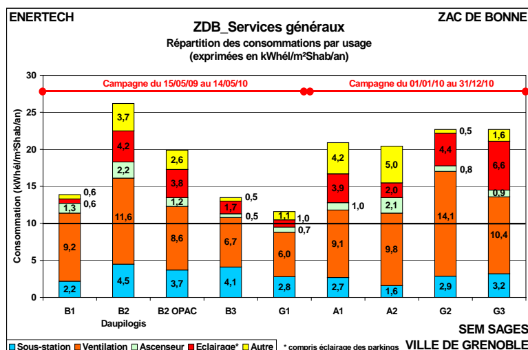
Figure 19 : Consommation électrique des parties communes
