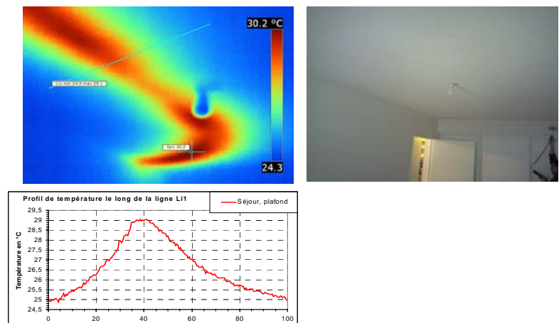
Figure 10 : Photographie infrarouge d'un plafond de logement
