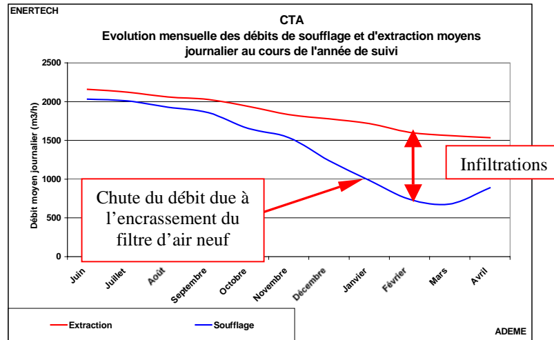
Figure 12 : Evolution des débits moyens journaliers dans une installation double flux
