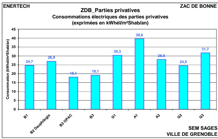
Figure 26 : Consommations électrodomestiques (moyenne des logements suivis dans chaque bâtiment) exprimées en kWh él /m 2 Shab/an
