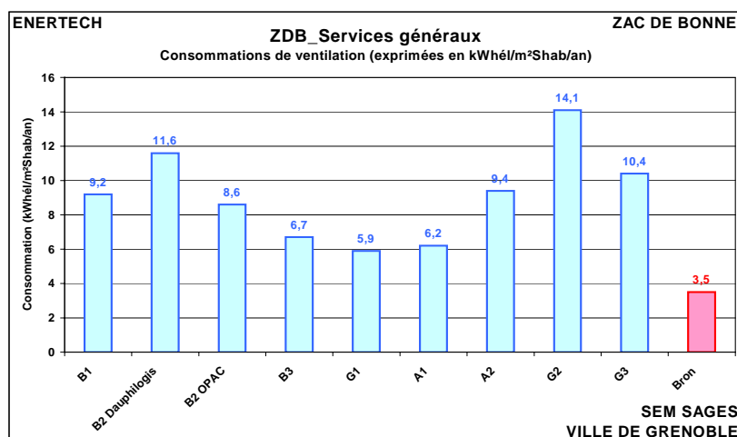
Figure 15 : Consommations électriques des installations de ventilation
