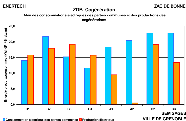
Figure 28 : Consommations des cogénérations
